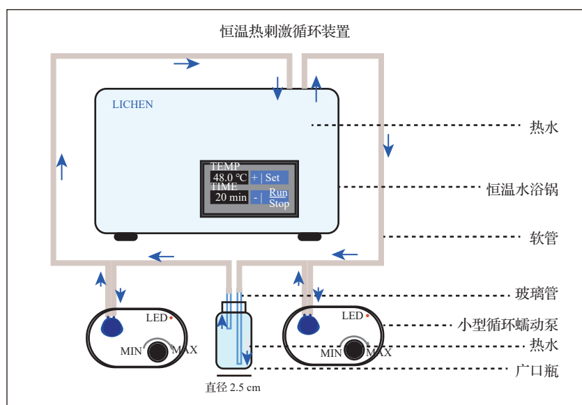
图1 热刺激恒温循环干预装置示意图
